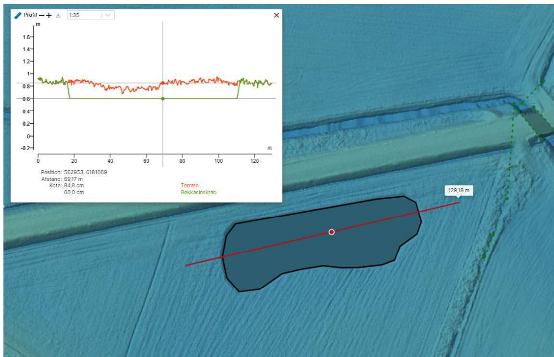
Figur 4-5 Tværsnit fra Scalgo som viser bundkoten af bekkasinskrabet og terrænet før og efter etablering af skrabet.
